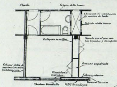
Habitación tipo de esta planta. Escala 1:50.
